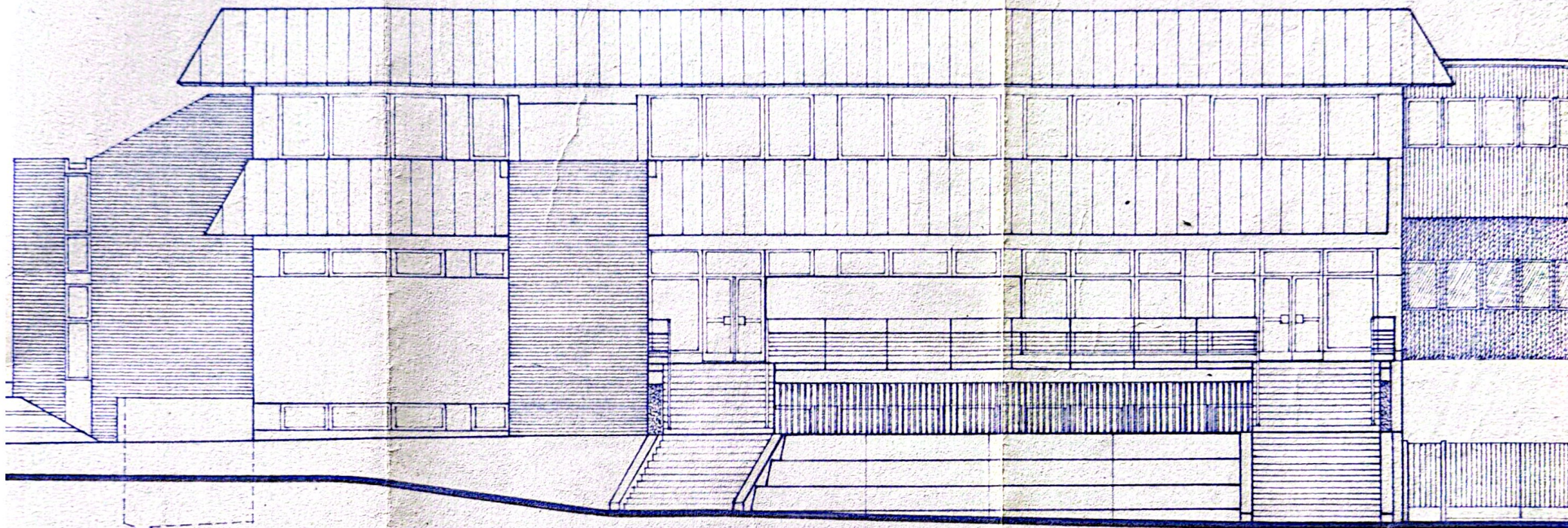
BUDYNEK DOM TECHNIKA ELEWACJA PÓŁNOCNA SKALA 1:100
